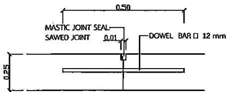
LONGITUDINAL JOINT
