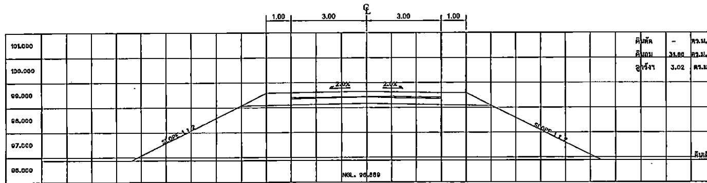
ผิวจราจรคอนกรีต 6.00 ม. ไหลทางลูกรังสองข้างทาง ละ 1.00 ม.
