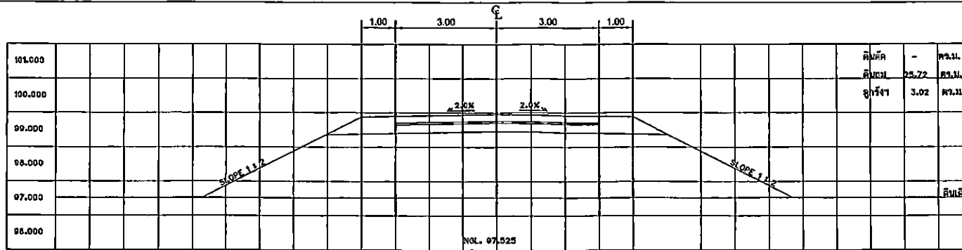
ผิวจราจรคอนกรีต 6.00 ม. ไหล่ทางลูกรังสูงข้างละ 1.00 ม.
