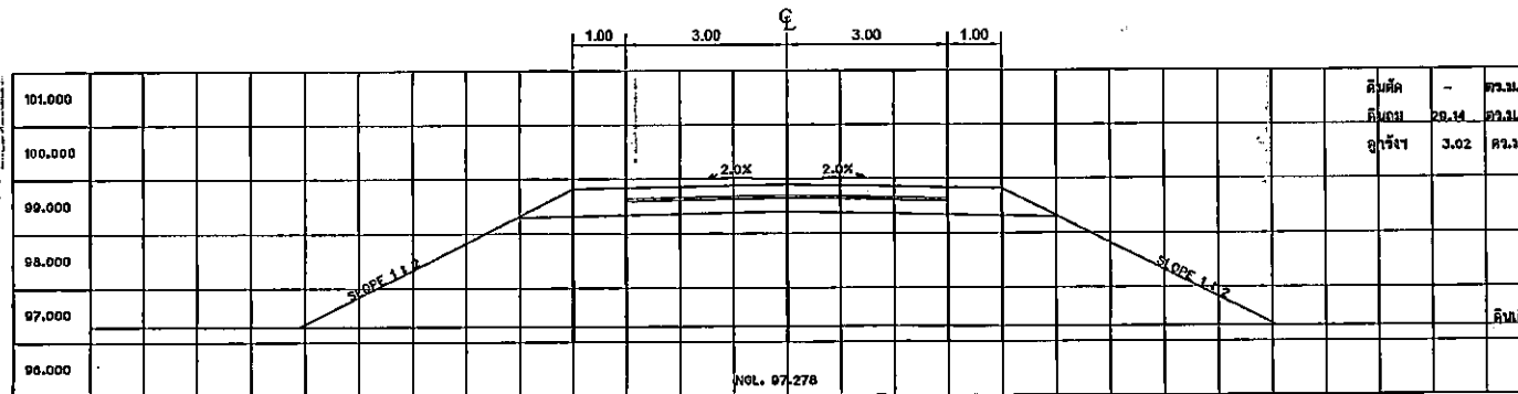
ผิวจราจรคอนกรีต ๓.๐๐ ม. ไหล่ทางลูกรังล้นข้างๆ ละ 1.๐๐ ม.
