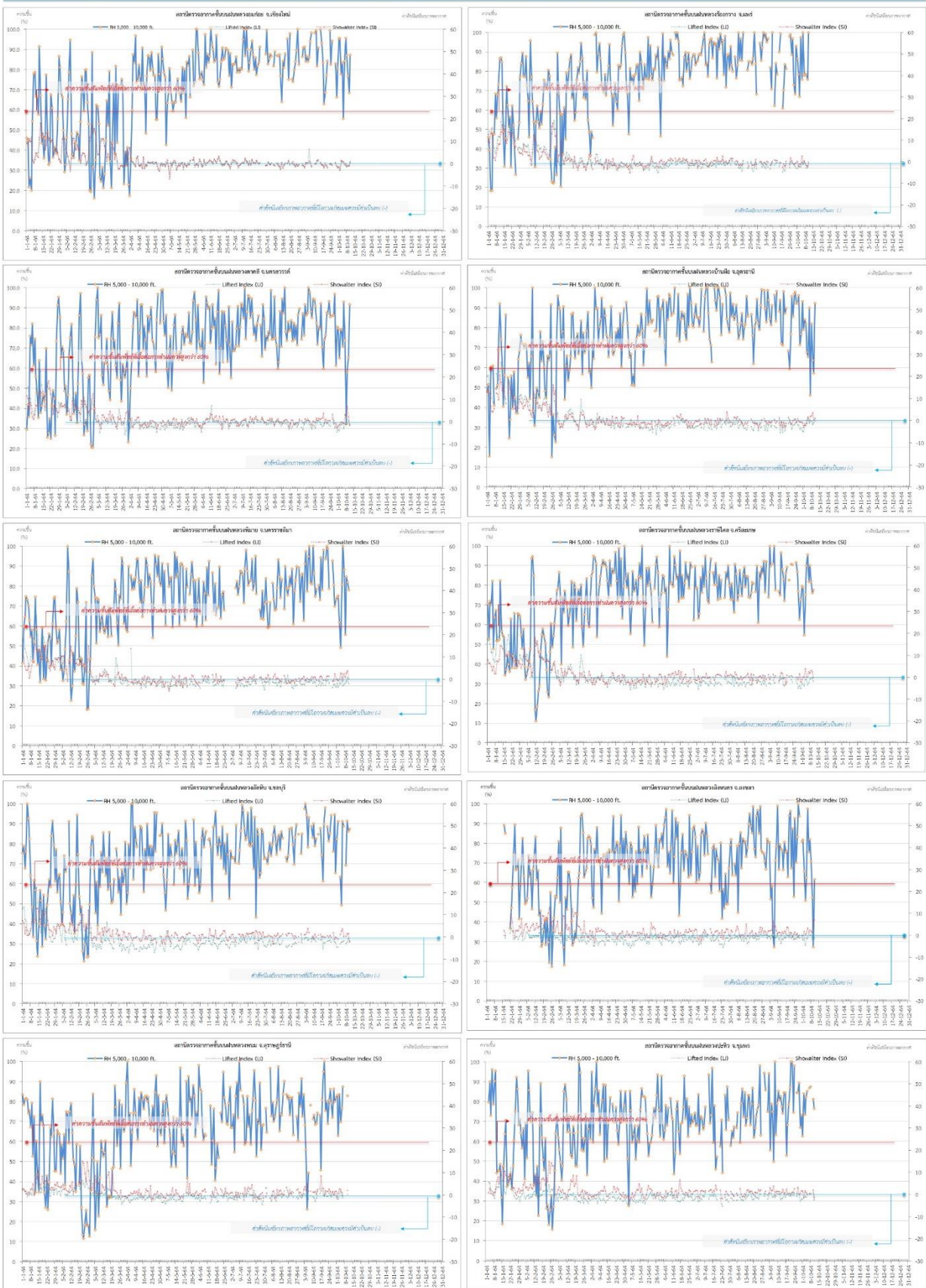
กราฟแสดงมลตรวจอากาศชั้นบน (ระยะ 5,000 - 10,000 ฟุต) ตั้งแต่วันที่ 1 มกราคม 2564 - ปัจจุบัน
