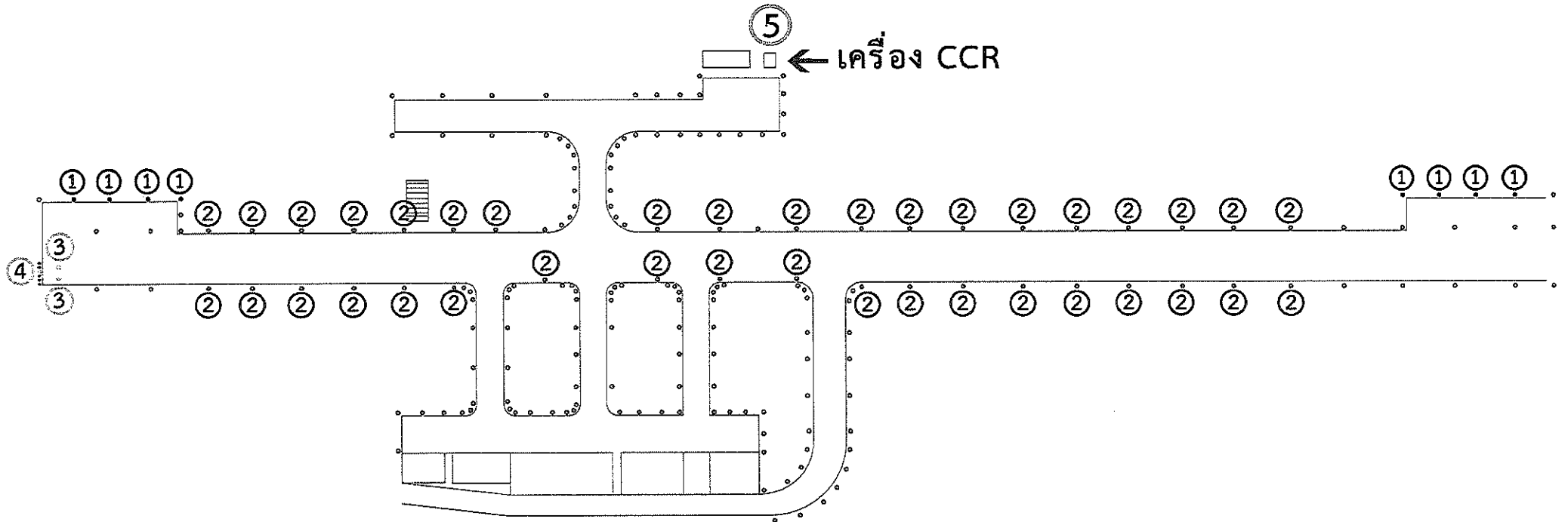
แผนผังแสดงจุดปรับปรุงระบบไฟฟ้าทางวิ่งและทางขับอากาศยาน (Runway, Threshold/END, Taxiway & Turd PAD)
